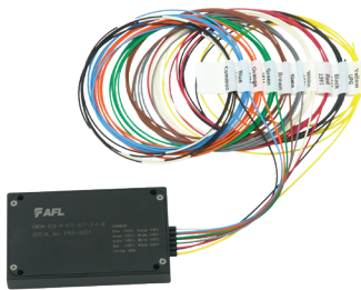
CWDM 8-Channel Mini Module
